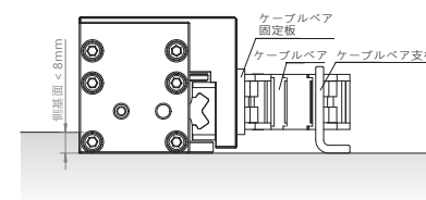
ケーブルベアを水平にセッティングする1
