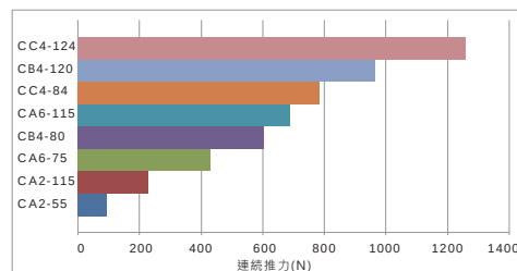
C-series 鉄心式連続推力一覧表
