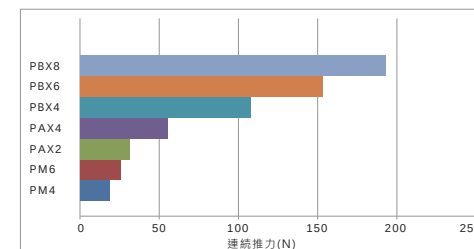
P-series 無鉄心式連続推力一覧表
