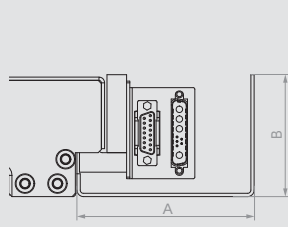
H-横型チェーン
