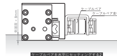
ケーブルベアを水平にセッティングする2
