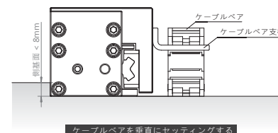
ケーブルベアを垂直にセッティングする
